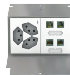
3xT13 + 2x 2xRJ45
