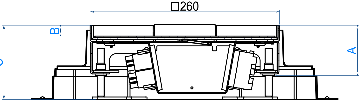
Ansicht mit Einbaubox
